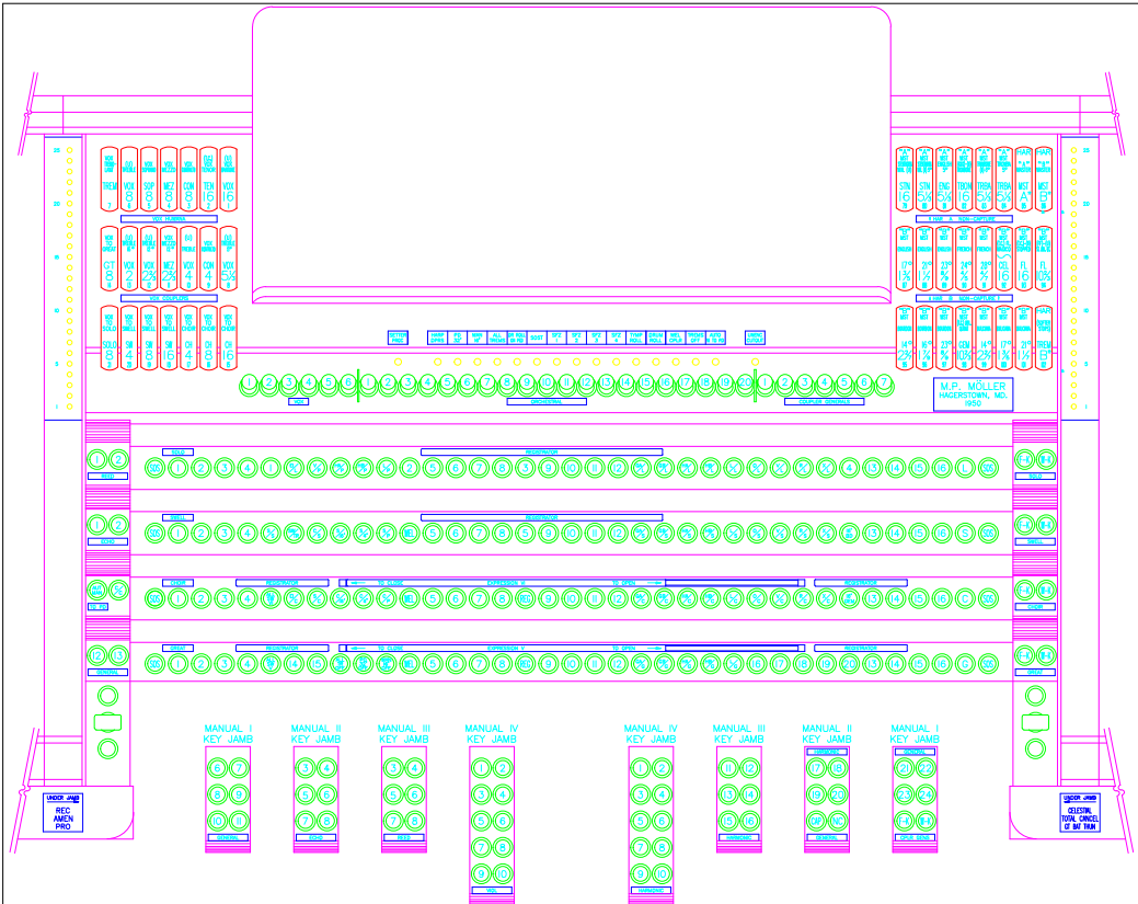
SCALE: 6" = 1'-0"
